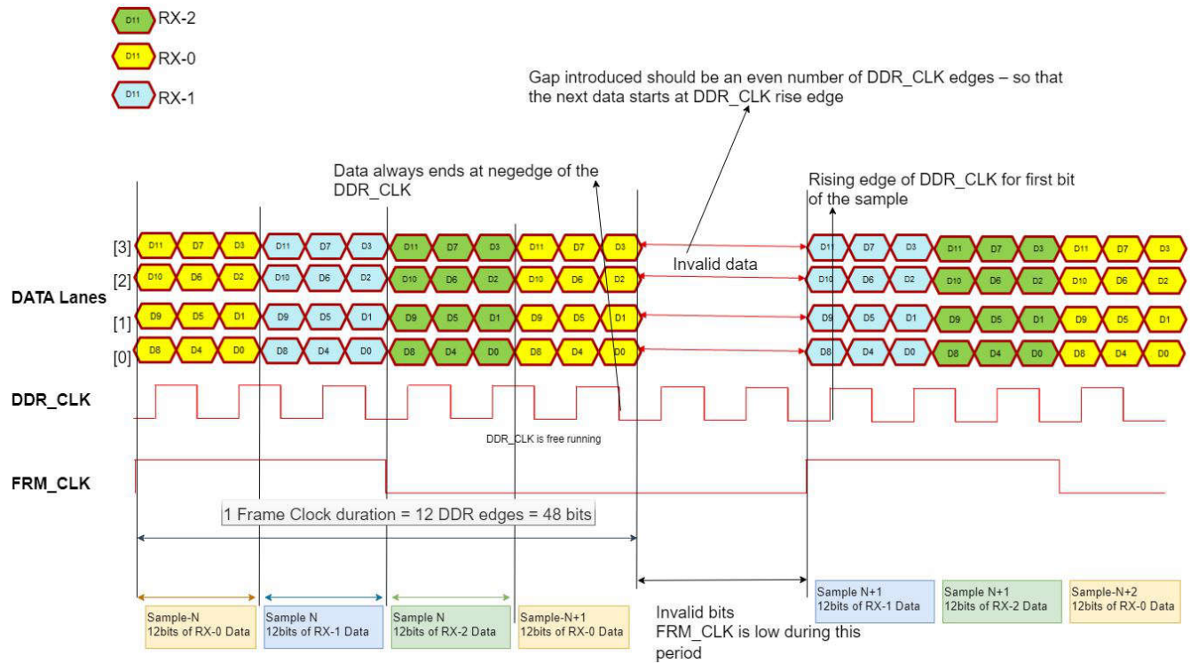
Figure 8-14. RDIF Data Format
